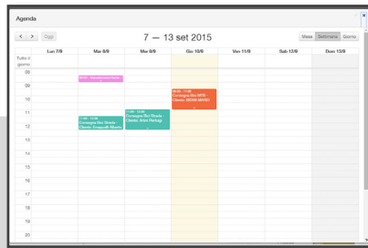
schermata AGENDA
