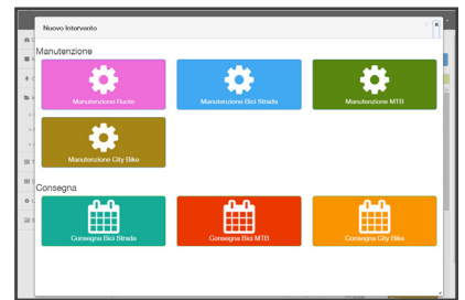
schermata INTERVENTI
