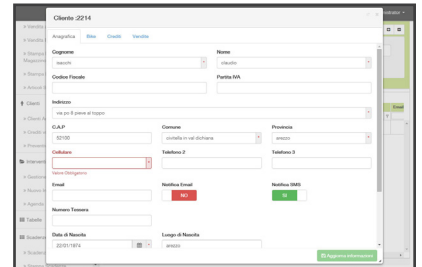
schermata CLIENTI
